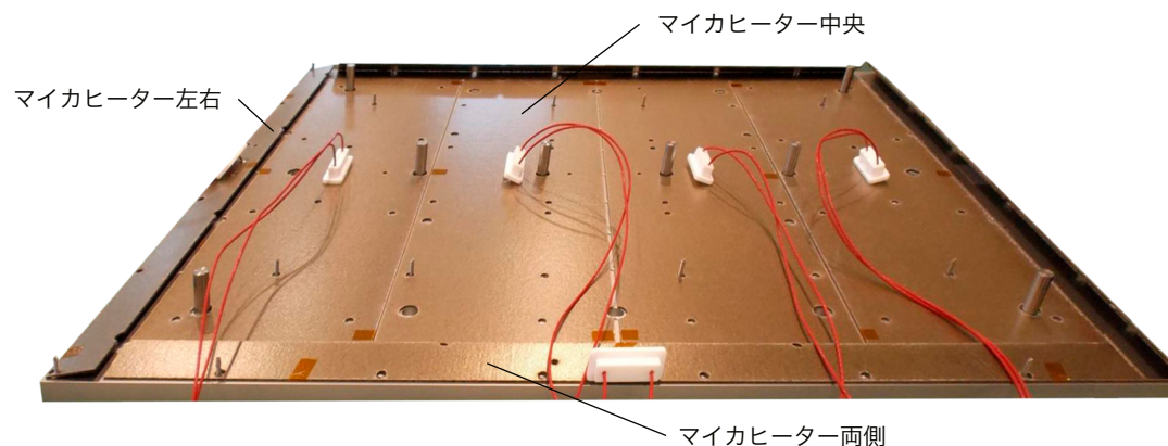
Heater Plateを裏から見た写真です。中央 4枚 両側 1枚ずつ左右1枚ずつの8分割Heaterです。
